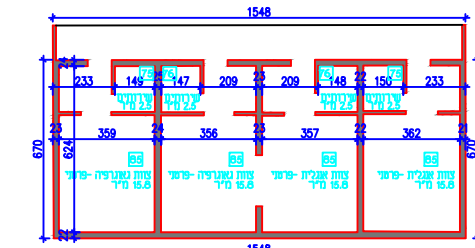
תכנית מבנה מס 13 - צוות אנגלית - 835
